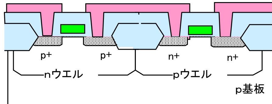
(c) ツインタブ型 (ツインウエル型)
