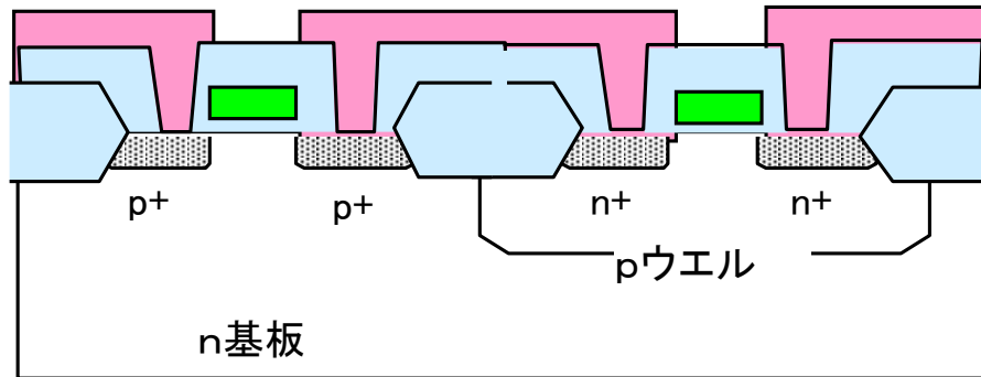
(a) pウエル型
